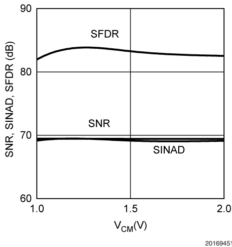
SNR, SINAD, SFDR vs. V_{CM}
